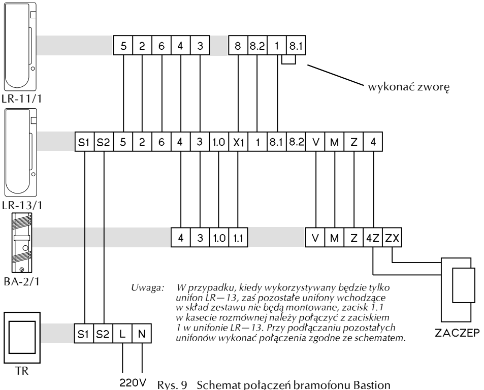
Rys. 9 Schemat połączeń bramofonu Bastion z jednoprzyciskową kasetą rozmówną i dwoma unifonami z łącznością wewnętrzną
