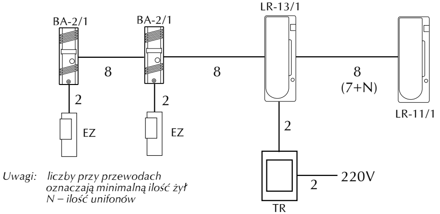
Rys. 8 Schemat blokowy połączeń bramofonu Bastion z dwiema jednoprzyciskowymi kasetami rozmównymi i dwoma unifonami z łącznością wewnętrzną
