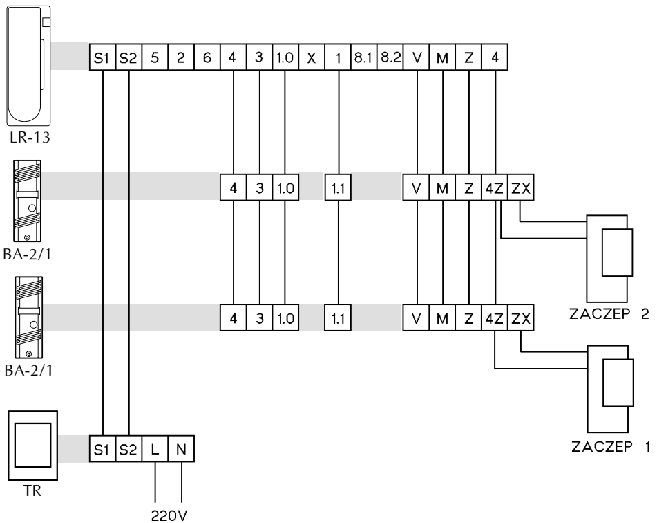
Rys. 9 Schemat połączeń bramofonu Bastion z dwiema kasetami rozmównymi i jednym unifonem
