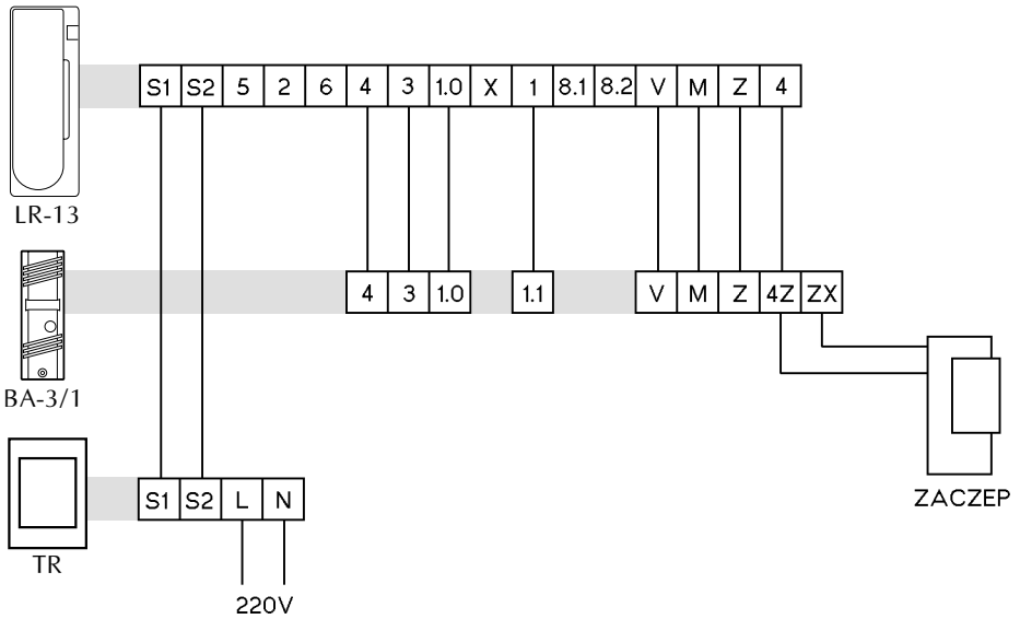
Rys. 9 Schemat połączeń bramofonu Bastion z jedną kasetą rozmówną i jednym unifonem
