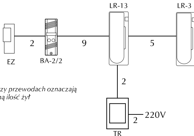
Rys. 8 Schemat blokowy połączeń bramofonu Bastion z jedną dwuprzyciskową kasetą rozmówną i dwoma unifonami bez łączności wewnętrznej
