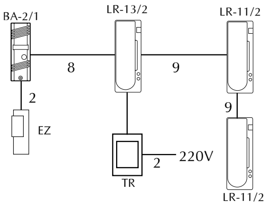
Rys. 8 Schemat blokowy połączeń bramofonu Bastion z jedną jednoprzyciskową kasetą rozmównymi i trzema unifonami z łącznością wewnętrzną
