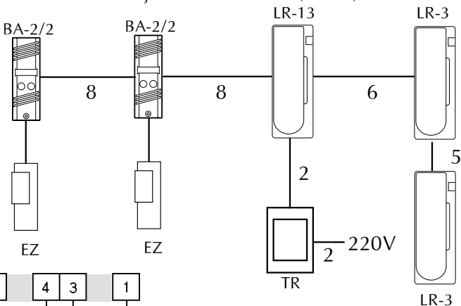
Rys. 8 Schemat blokowy połączeń bramofonu Bastion z dwuprzyciskowymi kasetami rozmównymi i trzema unifonami bez łączności wewnętrznej
