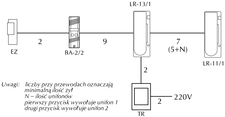
Rys. 8 Schemat blokowy połączeń bramofonu Bastion z dwuprzyciskową kasetą rozmówną i dwoma unifonami z łącznością wewnętrzną
