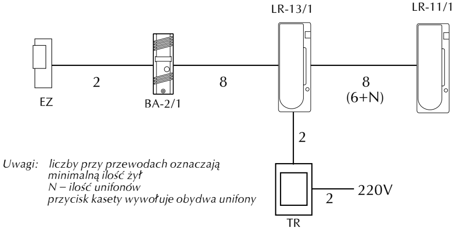
Rys. 8 Schemat blokowy połączeń bramofonu Bastion z jednoprzyciskową kasetą rozmówną i dwoma unifonami z łącznością wewnętrzną
