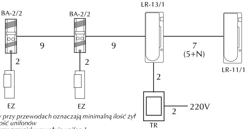
Rys. 8 Schemat blokowy połączeń bramofonu Bastion z dwiema dwuprzyciskowymi kasetami rozmównymi i dwoma unifonami z łącznością wewnętrzną
