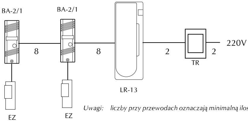
Rys. 8 Schemat blokowy połączeń bramofonu Bastion z dwiema kasetami rozmównymi i jednym unifonem
