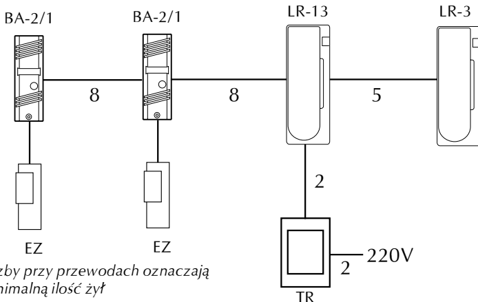
Rys. 8 Schemat blokowy połączeń bramofonu Bastion z dwiema jedнопrzyciskowymi kasetami rozmównymi i dwoma unifonami bez łączności wewnętrznej
