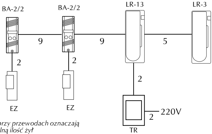
Rys. 8 Schemat blokowy połączeń bramofonu Bastion z dwiema dwuprzyciskowymi kasetami rozmównymi i dwoma unifonami bez łączności wewnętrznej
