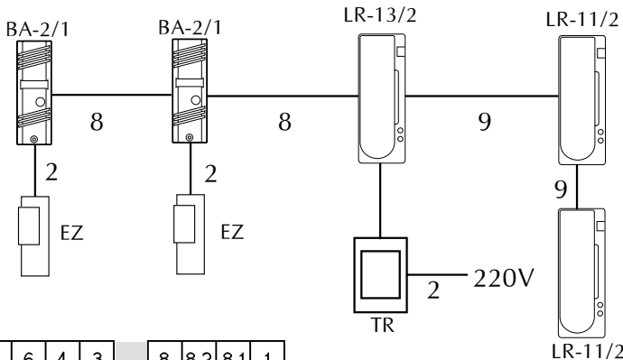
Rys. 8 Schemat blokowy połączeń bramofonu Bastion z dwiema jedнопrzyciskowymi kasetami rozmównymi i trzema unifonami z łącznością wewnętrzną
