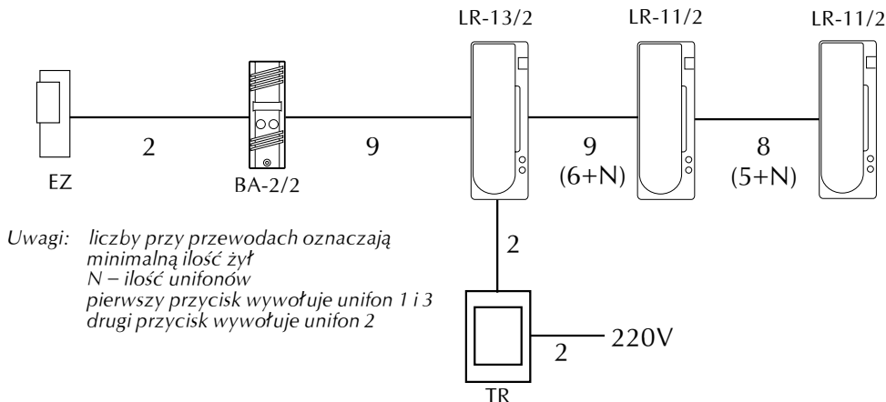
Rys. 8 Schemat blokowy połączeń bramofonu Bastion z dwuprzyciskową kasetą rozmówną i trzema unifonami z łącznością wewnętrzną
